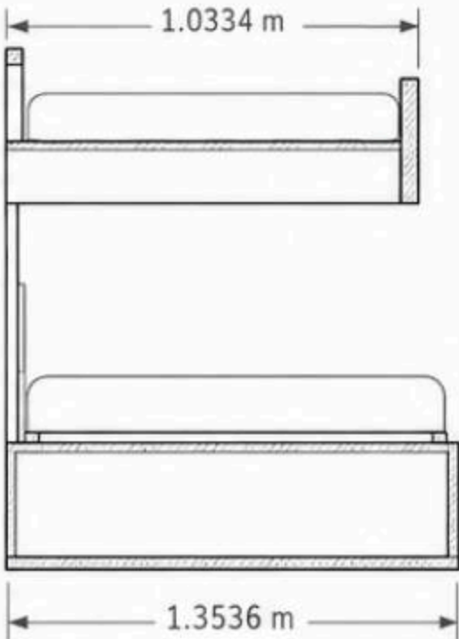
VISTA LATERAL / SECCIÓN TRANSVERSAL
