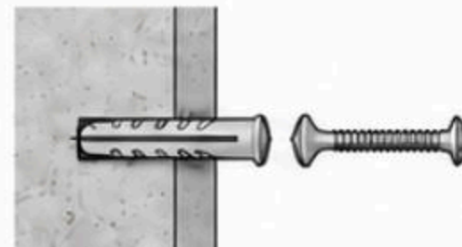
TAQUETE Y TORNILLO OCULTO (anclaje a muro y piso)
